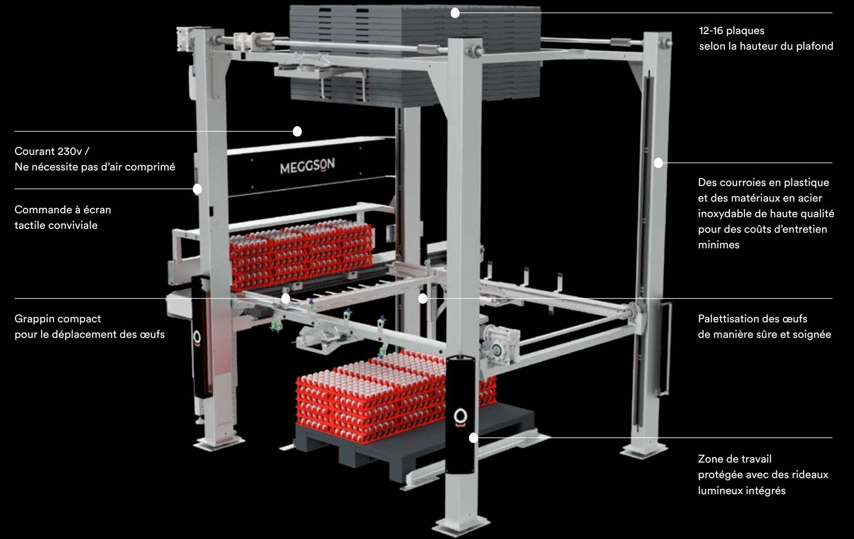
Caractéristiques du Meggbot TP100
